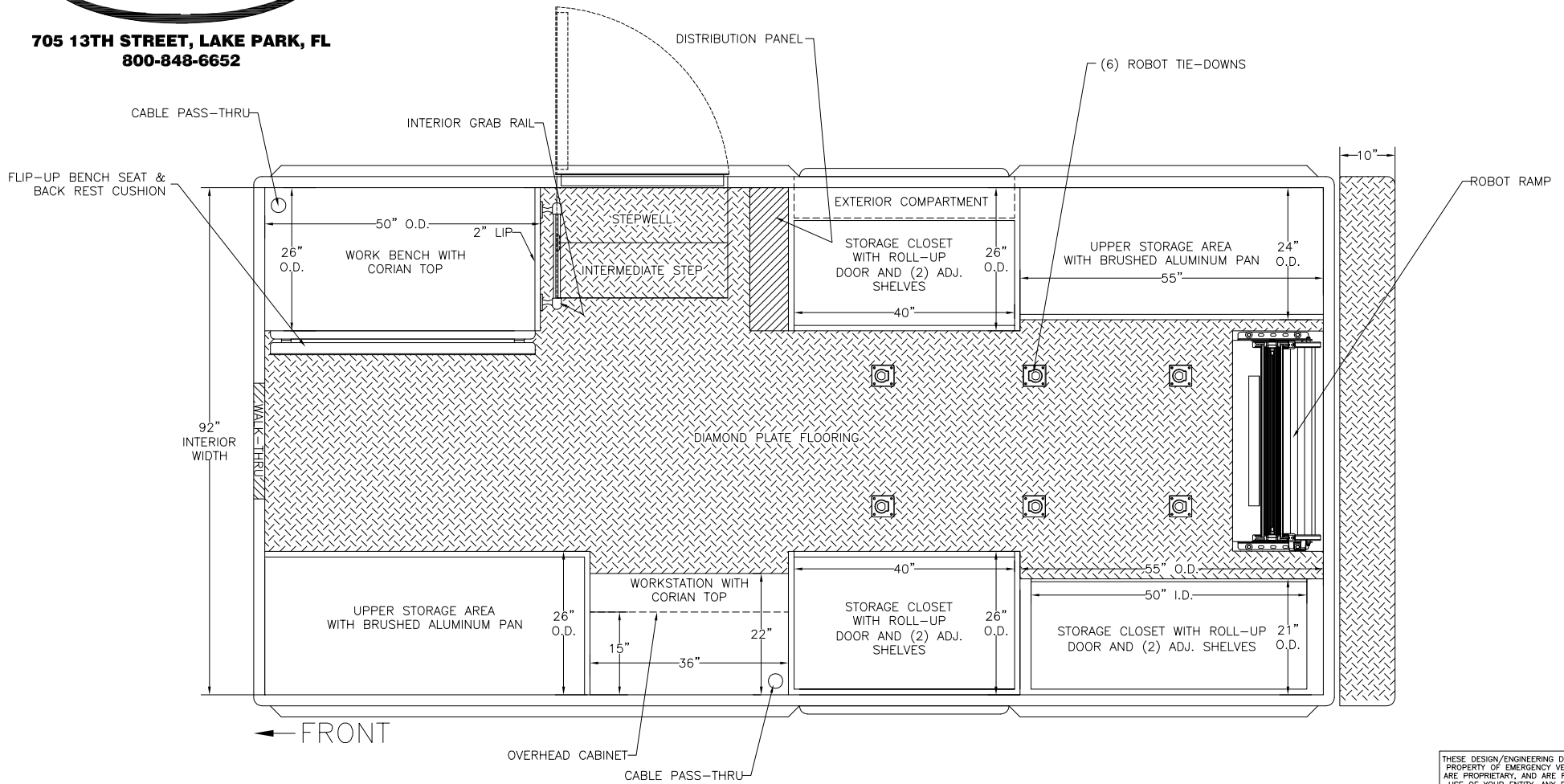
Body Planview
